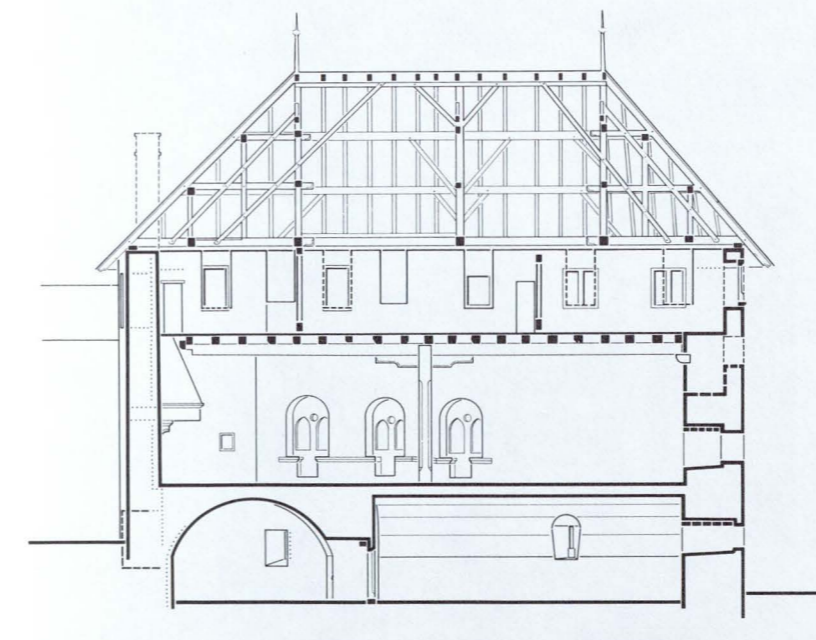
Längsschnitt durch den Palas gegen Süden. Über dem Rittersaal die zum Teil in Fenster umgewandelte Zinnenreihe des 14. Jh. und der Dachstuhl von 1395. Pläne: Othmar Mabboux.
