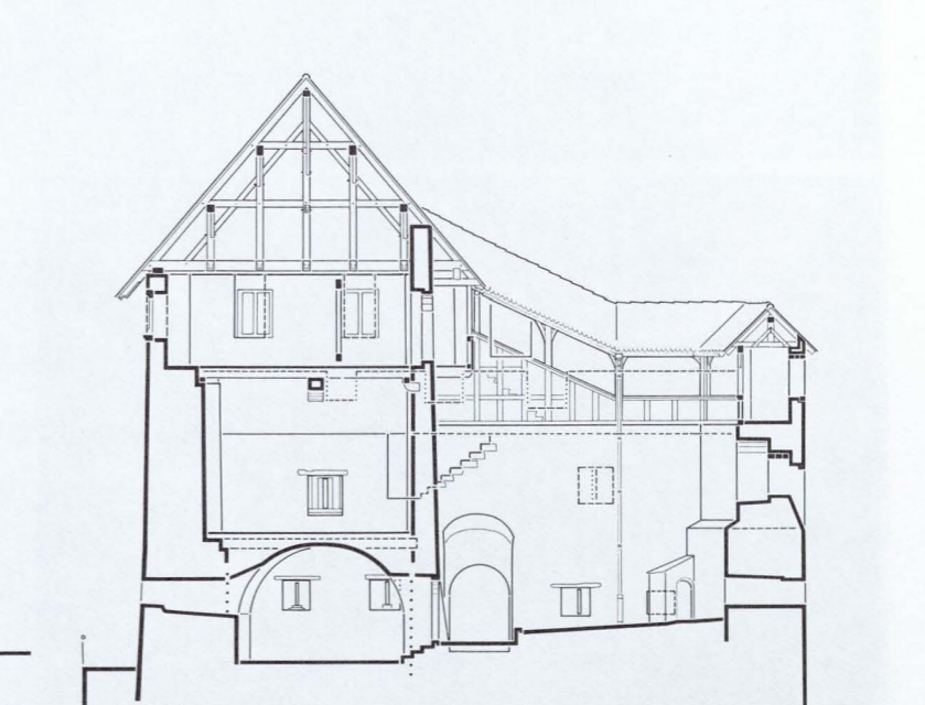
Querschnitt durch Palas und Hof gegen Westen. In den abnehmenden Mauerstärken der Nord- und Südmauer sind Konstruktionsetappen abzulesen. In der Westmauer eingetragen ältere Zinnen- und Schartensysteme.
